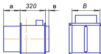
Рис. 2. Общий вид клапана с электромеханическим приводом.
