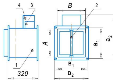
Рис.1. Установочные, габаритные и размеры внутреннего сечения клапана.
