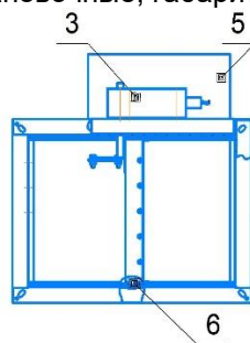
Рис. 2. Общий вид клапана с электромеханическим приводом.
