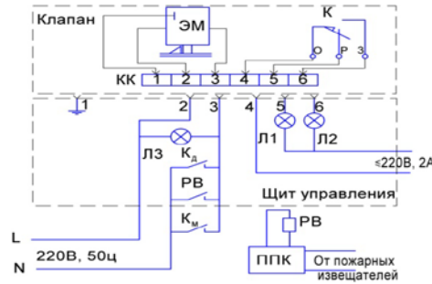
Рис. 4. Примеры схем установки клапана различных исполнений
