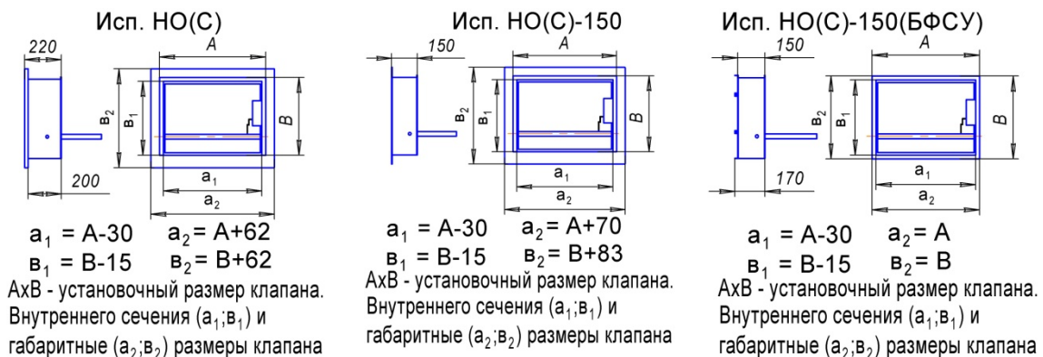
Рис.1. Установочные, габаритные и размеры внутреннего сечения клапана.
