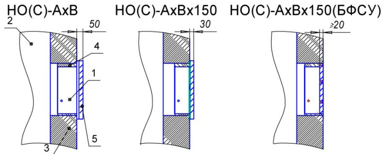
Рис. 4. Примеры схем установки клапана различных исполнений
