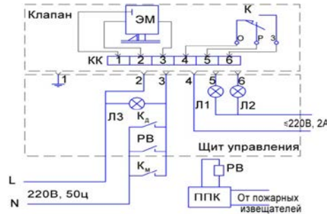
Рис. 4. Примеры схем установки клапана различных исполнений
