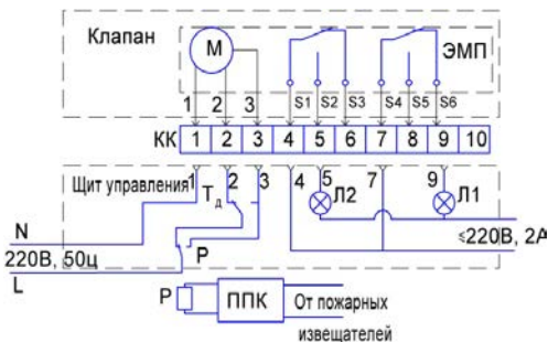
Рис.5а. Пример электрической схемы подключения клапана с электромеханическим приводом с возвратной пружиной.
