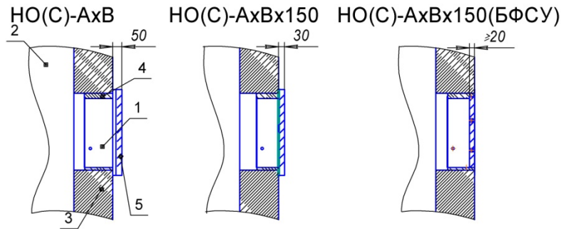
Рис. 4. Примеры схем установки клапана различных исполнений
