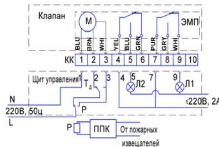
Рис.5а. Пример электрической схемы подключения клапана с электромеханическим приводом с возвратной пружиной.
