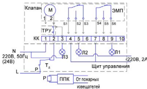
Рис. 5. Пример электрической схемы подключения клапана с электромагнитным приводом.
