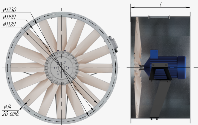
Габаритные и присоединительные размеры
